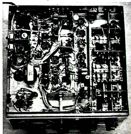
Bild 8. Chassisunteransicht des „R-4“
