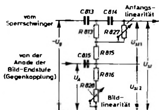
Bild 95. Prinzipschaltung der Korrektur der gesamten Bildlinearität
