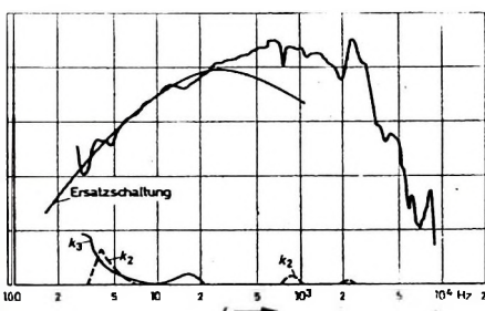
Bild 5. Frequenzgang der Grundwelle des Tieftonlautsprechers ohne Beschwerungsring und Frequenzgang seiner Ersatzschaltung; k_2 , k_3 Frequenzgänge der zweiten und dritten Harmonischen
