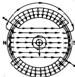
Bild 98. Vertikale Ablenkung des Elektronenstrahls der Bildröhre durch das Zusammenwirken des Magnetfeldes der Bildablenkspulen (Toroidspulen) und des Magnetfeldes des Elektronenstrahls
