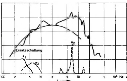
Bild 4. Frequenzgang der Grundwelle des Tieftonlautsprechers mit Beschwerungsring und Frequenzgang seiner Ersatzschaltung; k_2 , k_3 Frequenzgänge der zweiten und dritten Harmonischen
