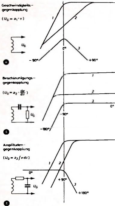
Bild 8. Wirkung von Gegenkopplungen („Motivational Feedback“)
