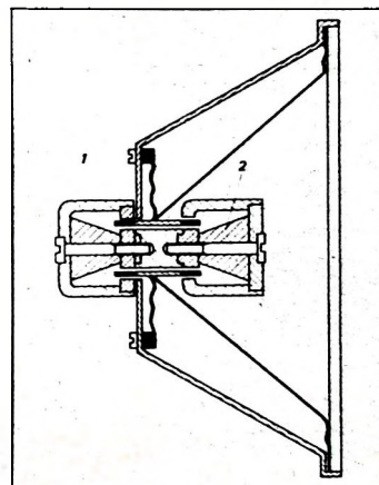
Bild 7. Lautsprecher mit Gegenkopplungssystem
