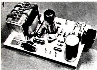
▲ Bild 1. Gesamtansicht der Gegenakt-Endstufe
