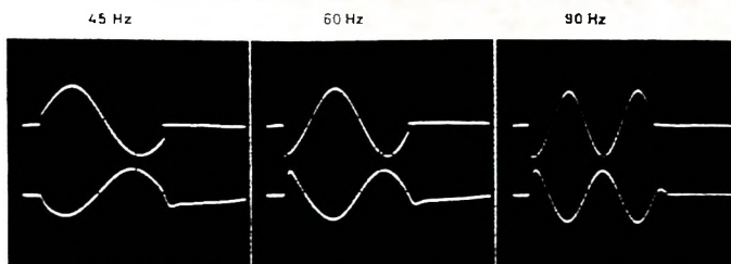
Bild 6. Einschwingverhalten der Ersatzschaltung eines Tieftonlautsprechers mit Entzerrung; oben Eingangsspannung, unten Ausgangsspannung
