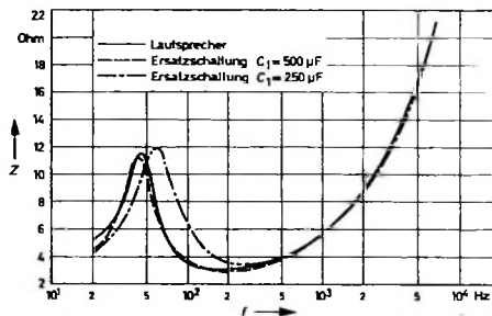
Bild 2. Impedanzverlauf eines Tieftönlautsprechers mit 25 cm Membrandurchmesser und von Ersatzschaltungen des Lautsprechers
