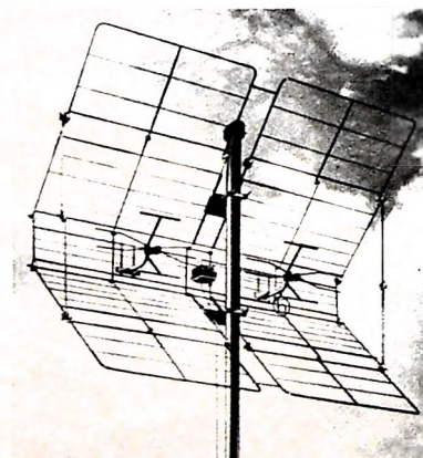
Winkelreflektor-Zweibereichantenne „Fesa Corner 6“ von Hirschmann
