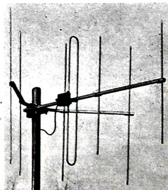
Vertikal polarisierte Kanalgruppenantenne „FV 7“ von R. Bosch Elektronik
