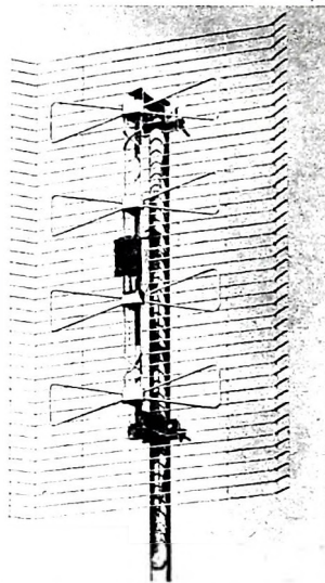
Siemens-Reflektorantenne „SAA 176“
