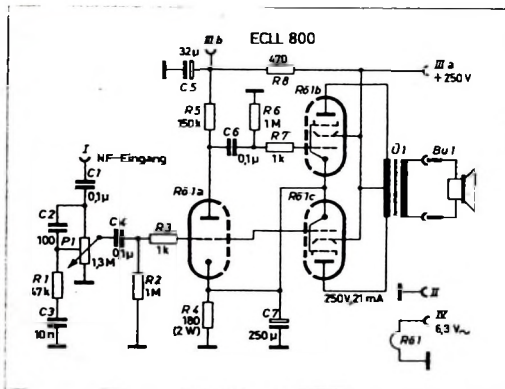
Bild 2. Schaltung des Gegentakl-Endstufen-Bausteins mit der ECLL 800
