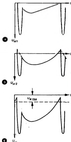
Bild 96. Entstehung der Steuerspannung U_{A1} : a) Anfangslinearität ( U_{A11} ), b) parabel förmige Vorverzerrung am Gegenkopplungsglied C_{815} , R_{816} , R_{828} ( U_{A12} ), c) Steuerspannung U_{A1} = U_{A11} + U_{A12} am Gitter 1 der Bild-Endröhre
