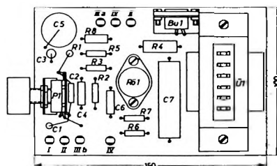
Bild 3. Einzelteileanordnung
